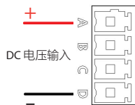
0-100V电压信号输入
