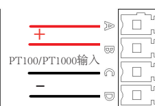
4线制PT100/PT1000信号输入
