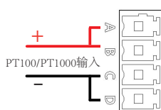
2线制PT100/PT1000信号输入
