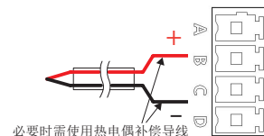
热电偶信号输入
