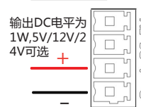
DC 电平输出
