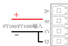
3线制PT100/PT1000信号输入
