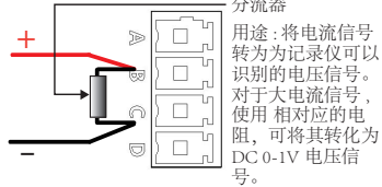
大电流信号输入
