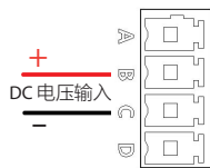
0-1V电压信号输入
